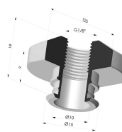
Inserto fêmea removível 1/8G
