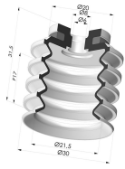
Ventosa 4.5 Fole Série 92 Ø 30MM
