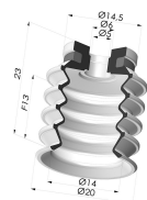
Ventosa 4.5 Fole Série 92 Ø 20MM
