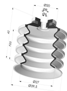
Ventosa 4.5 Fole Série 92 Ø 40MM
