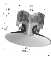
Ventosa plana Série 9 Ø 31,5 mm
