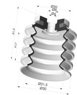
Ventosa 4.5 Soffietti Serie 92 Ø 30MM
