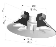
Ventosa Piatta Serie 90 Ø 53MM
