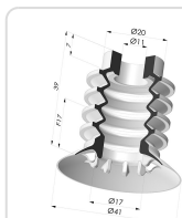
Ventosa 4.5 Soffietti Serie 95 Ø 41MM
