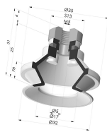
Ventosa 1.5 Soffietti Serie 91 Ø 31,8MM
