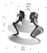
Ventosa 1.5 Soffietti Serie 91 Ø 22,2MM
