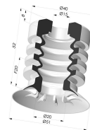
Ventosa 4.5 Soffietti Serie 95-2 Ø 51MM
