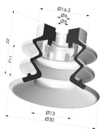
Ventosa 2.5 Soffietti Serie 96C Ø 30MM
