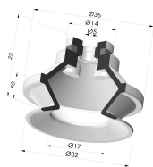
Ventouse 1.5 Soufflets Série 91 Ø 31,8MM
