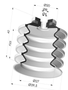
Ventouse 4.5 Soufflets Série 92 Ø 40MM
