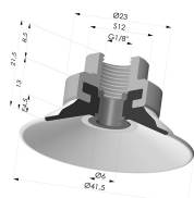
Ventouse Plate Série 9 Ø 41,5MM
