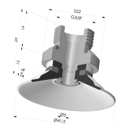
Ventouse Plate Série 9 Ø 41,5MM
