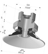
Ventouse Plate Série 9 Ø 41,5MM
