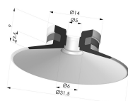
Ventouse Plate Série 9 Ø 31.5MM
