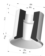
Ventouse Plate Série 9 Ø 11MM
