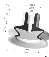
Ventouse 1.5 Soufflets Série 8A Ø 49MM
