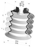
Ventosa 4.5 Fuelles Serie 92 Ø 50MM
