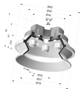
Ventosa 1.5 Fuelles Serie 91 Ø 75MM
