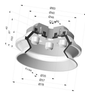
Ventosa 1.5 Fuelles Serie 91 Ø 75MM
