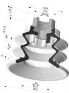
Ventosa 2.5 Fuelles Serie 96C Ø 70MM
