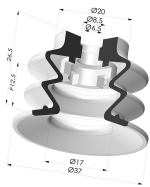
Sauggreifer 2.5 Falten Serie 96 Ø 35MM
