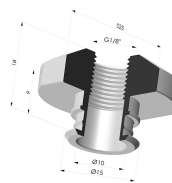
Abtrennbarer Halter IG 1/8G
