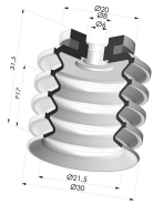
Sauggreifer 4.5 Falten Serie 92 Ø 30MM
