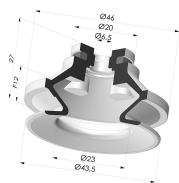
Sauggreifer 1.5 Falten Serie 91 Ø 40MM
