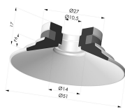
Flachsauggreifer Serie 9 Ø 51MM
