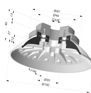
Flachsauggreifer Serie 94 Ø 100MM
