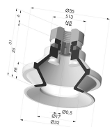
Sauggreifer 1.5 Falten Serie 91 Ø 31.8MM
