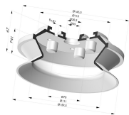
Sauggreifer 1.5 Falten Serie 91 Ø 159,5MM
