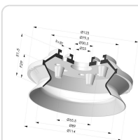
Sauggreifer 1.5 Falten Serie 91 Ø 114MM Produktreferenz: 91 110-- A
