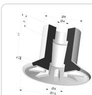
Flachsauggreifer Serie 90 Ø 16.5MM Produktreferenz: 90 15-- A
