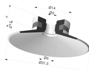
Flachsauggreifer Serie 9 Ø 31.5MM
