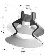
Sauggreifer 1.5 Falten Serie 8A Ø 44MM
