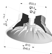
Flachsauggreifer Serie 99 Ø 40.5 mm
